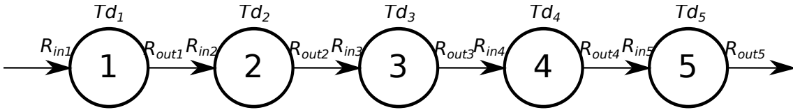
Figure 4.1 – Exemple d'un graphe SDF simple formé par 5 acteurs.
