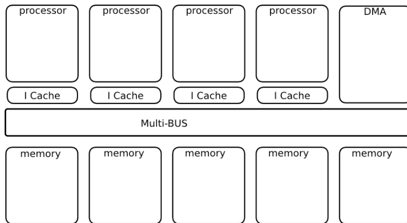
Figure 5.1 – Schéma bloc simplifié des premiers modules de l’architecture multi-cœurs pour le mobile proposé. Les processeurs sont connectés avec les bancs mémoires via un réseau de type multi-bus. Des modules DMA permettent une copie des données depuis et vers l’extérieur.
