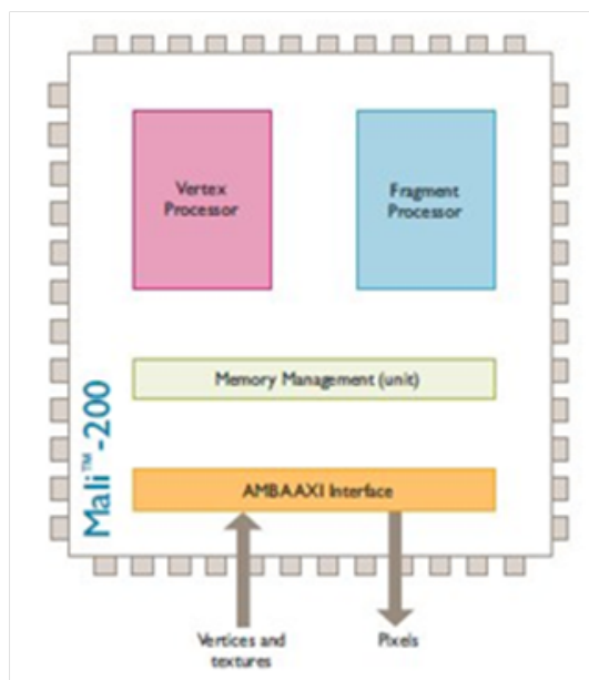
Figure 2.12 – L'architecture du GPU ARM Mali.
