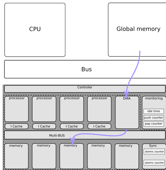
Figure 5.14 – Transfert de données depuis l'extérieur.
