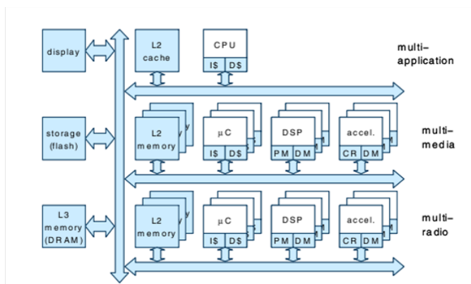
Figure 1.2 – Schéma d'une architecture mobile [5].
