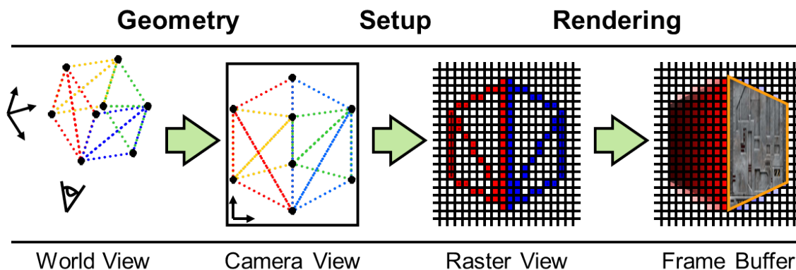
Figure 3.18 – Découpage du pipeline graphique en cinq parties, les données qui transitent entre la première et la deuxième partie sont des sommets ( v_0, v_1 ), puis des triangles ( t_0, t_1 ) entre la deuxième et la troisième partie, puis des tuiles ( b_0, b_1 ) entre les trois dernières parties.
