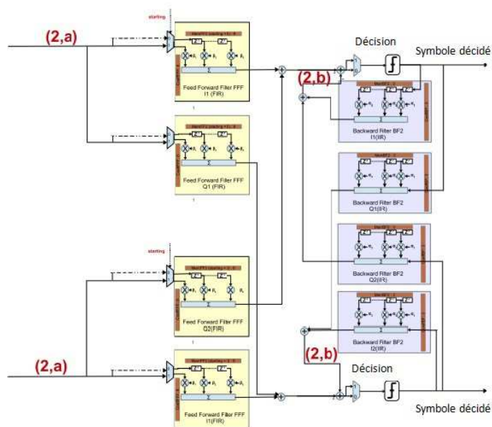
FIGURE 3.10 – Architecture d'un égaliseur DFE à coefficients complexes
