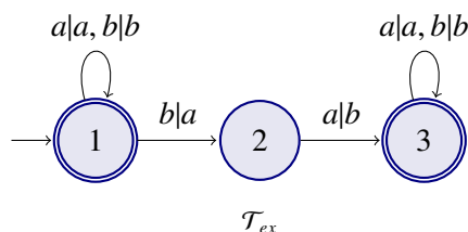
FIGURE 2.9 – \mathcal{T}_{ex} (Exemple de transducteur)
