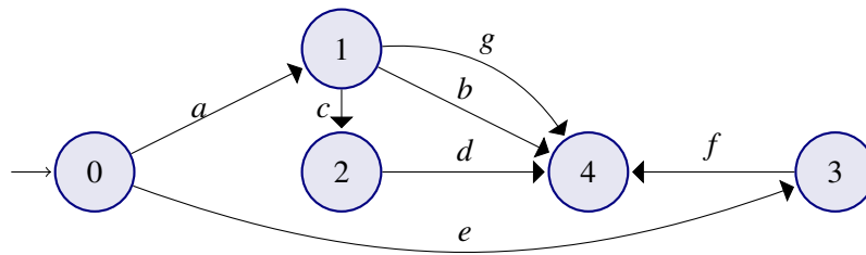
FIGURE 7.2 – Exemple de graphe fini
