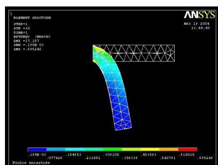
FIG. 4.5 – Résultats sous ansys : la poutre à l'état au repos, et à l'état d'équilibre (L'échelle de couleur indique le pourcentage de déformation, dans cette simulation, certains éléments sont à plus de 40% de déformation, ce qui est beaucoup)
