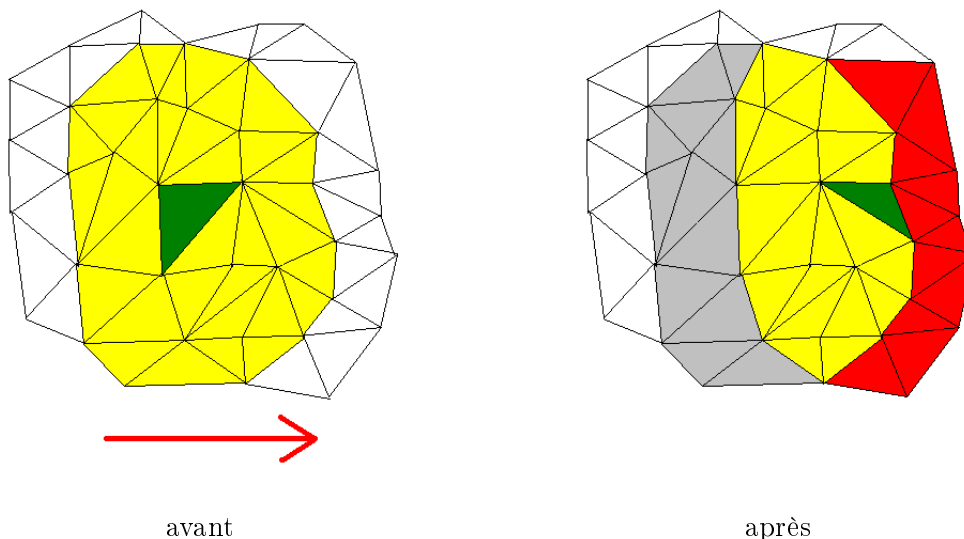
Figure 11 : Construction de la nouvelle région d'intérêt en utilisant la cohérence temporelle. On déplace vers la droite le centre d'intérêt (face verte), donc la région d'intérêt initiale (faces jaunes). Lors de la mise à jour, des faces sont enlevées : les faces grises ; des faces sont conservées : les faces jaunes ; et des faces sont ajoutées : les faces rouges. La nouvelle zone d'intérêt est donc constituée des faces jaunes et des faces rouges.
