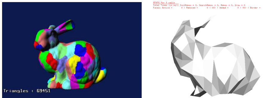
Figure 15.a : Clusterisation et maillage résultant pour un objet surfacique.
