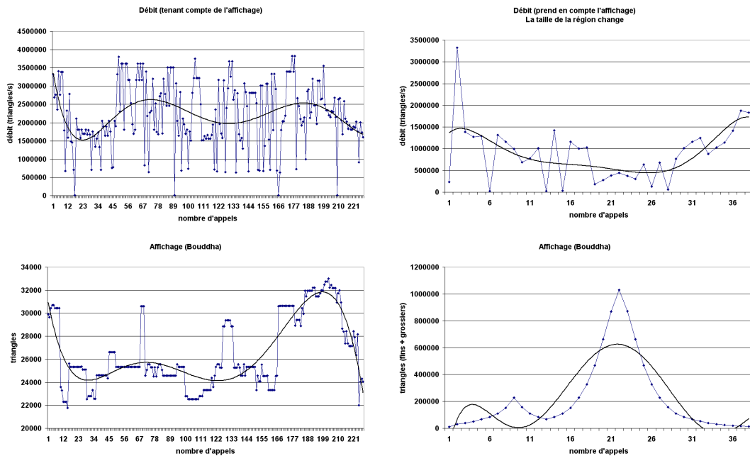
Figure 17.a : Courbes indiquant le nombre de triangles affichés en une seconde pour des maillages surfaciques. L'affichage est pris en compte dans les calculs.
