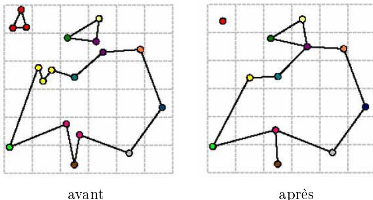
Figure 3 : Méthode de clusterisation avec une grille régulière.
