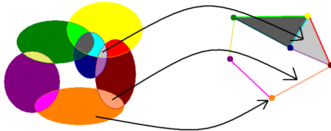
Figure 9 : Nerf associé à une collection de sous-ensembles.
