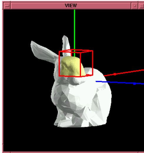
Figure 6 : Utilisation de MT avec une zone de focalisation cubique Le maillage est grossier en dehors de la boîte (en blanc) et fin dans la boîte (en jaune). Au niveau de la frontière, on trouve des triangles qui deviennent de plus en plus grossiers en s'éloignant. Cela est dû aux relations de dépendances entre les opérations de raffinement qui forcent certains dédoublements de sommets qui ne se trouvent pas dans la zone de focalisation.
