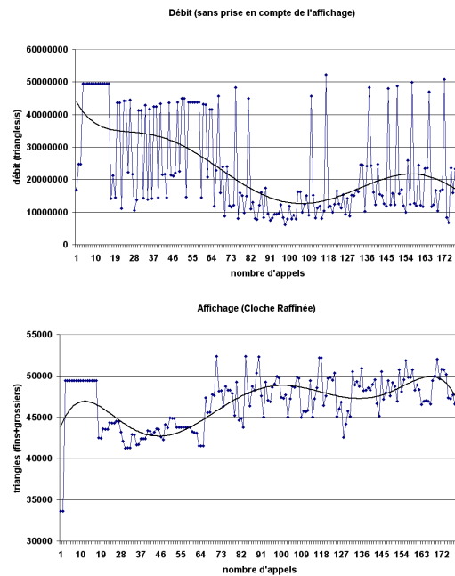
Figure 17.b : Courbes indiquant le nombre de triangles affichés en une seconde pour des maillages volumiques. L'affichage n'est pas pris en compte dans les calculs.
