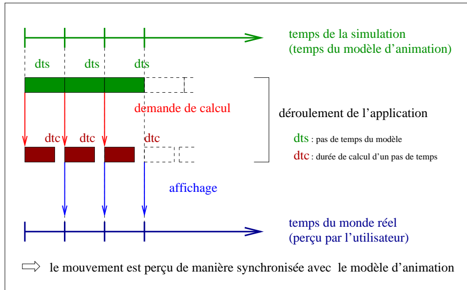
FIG. 3.3 – Dérroulement d'une simulation en temps réel
