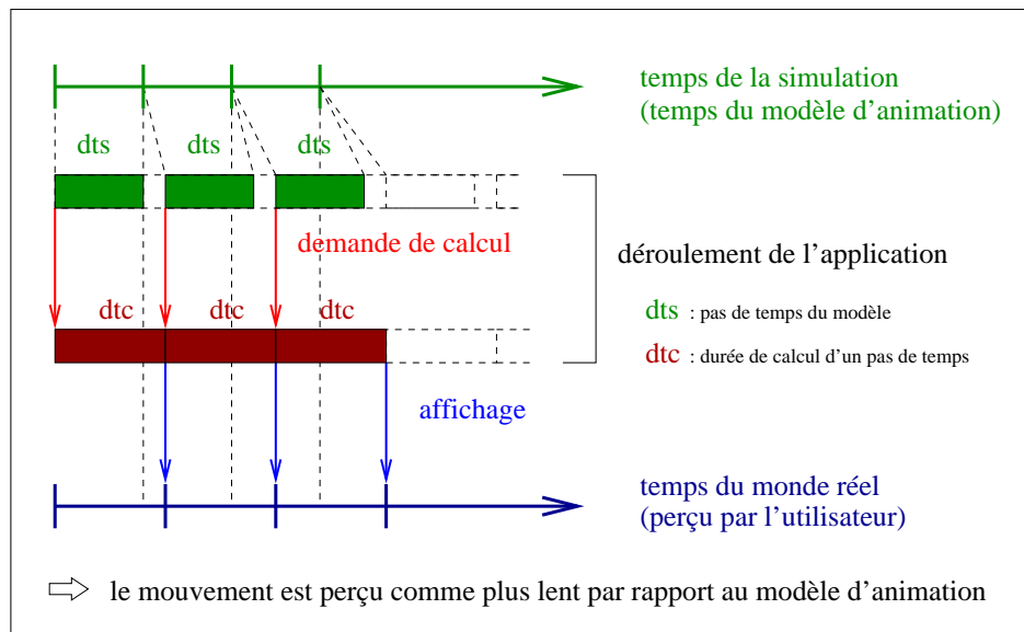
FIG. 3.4 – Dérroulement d'une simulation en temps différé
