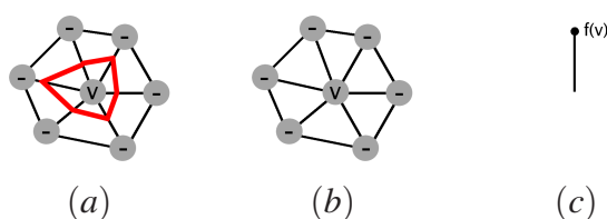
FIG. 2.6 – Ligne de niveau à proximité de v juste avant le passage de l’algorithme par v (a), et juste après (b), morceau rajouté au graphe après le passage par v (c).
