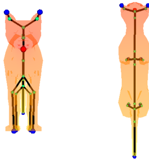
FIG. 4.7 – Mise en évidence de la symétrie du squelette.
