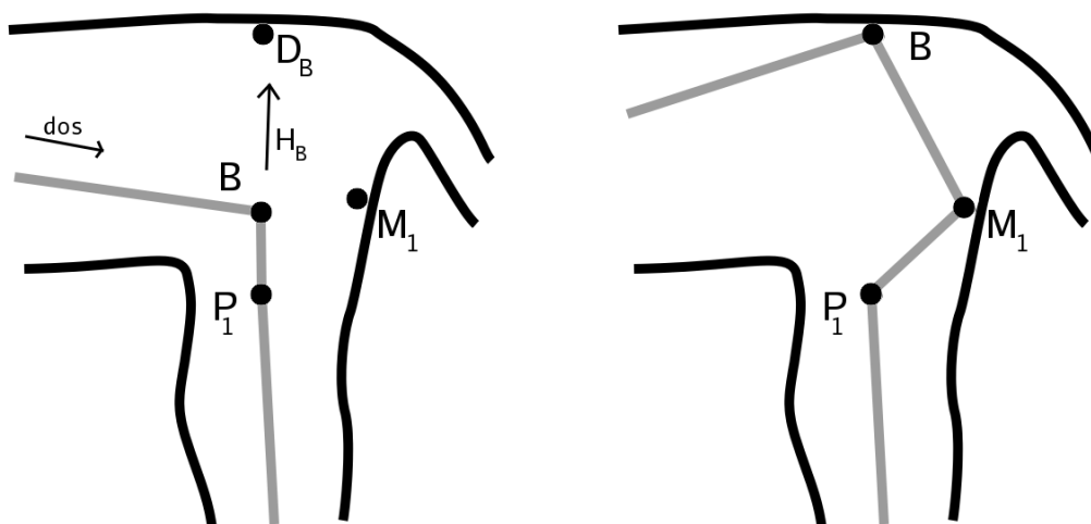
FIG. 5.4 – A gauche le squelette avant modifications et à droite le squelette modifié.
