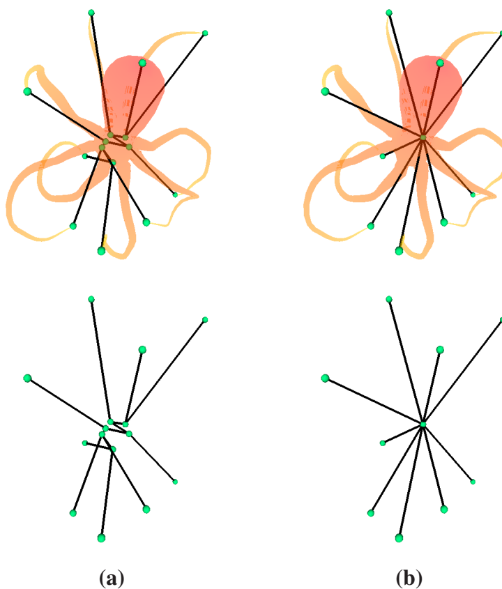
FIG. 3.5 – Graphe non symétrique obtenu à partir d'un modèle présentant une symétrie axiale (a), le même graphe obtenu en filtrant avec \beta = 0.007 , le nœud obtenu a une valence de 9 (b). Le graphe est simplifié au niveau des épaules et des mains.
