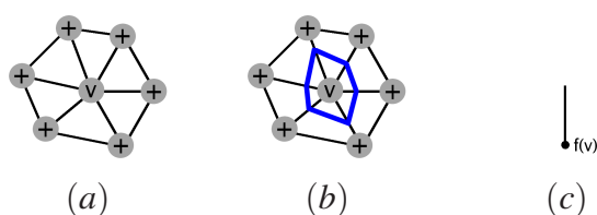
FIG. 2.4 – Ligne de niveau à proximité de v juste avant le passage de l’algorithme par v (a), et juste après (b), morceau rajouté au graphe après le passage par v (c).
