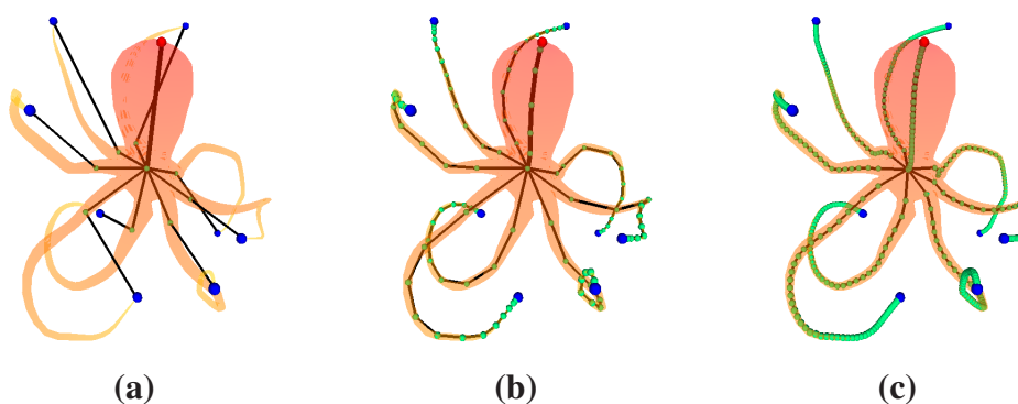
FIG. 4.12 – (a) : Le squelette après plongement en tenant compte de l'axe de rotation mais sans subdiviser. (b) et (c) : Le squelette après une subdivision plus ou moins fine des arêtes.
