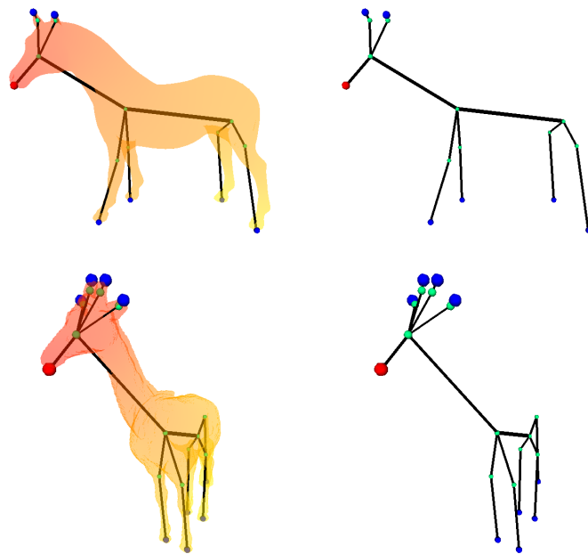
FIG. 4.15 – D’autres modèles et leurs squelettes.
