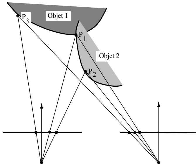
Figure 6.8. Lorsque deux points se trouvent sur la surface d'un objet peu incliné (1) l'ordre de leurs projections est le même dans les deux images. Si l'objet est fortement incliné (2) les projections ne sont pas vues simultanément dans les deux images si l'objet est opaque ou l'ordre est inversé si l'objet est transparent.
