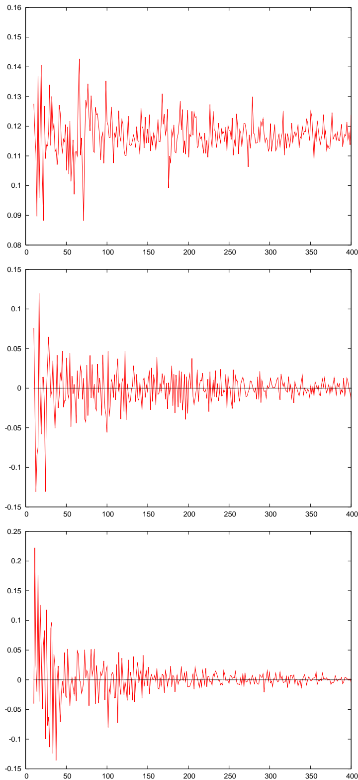
Figure 4. Top : \frac{k}{2\pi} \mapsto \frac{|U_{noisy}(k)|_{L^2(D)} - |U_{exact}(k)|_{L^2(D)}}{|U_{exact}(k)|_{L^2(D)}} . Middle : \frac{k}{2\pi} \mapsto \frac{|R_{est}(k)| - R|}{R} . Bottom : \frac{k}{2\pi} \mapsto \theta_i - \theta_{est}(k) .
