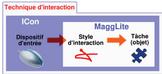
Figure 8 : Une technique d'interaction est définie par un dispositif d'entrée, un style d'interaction, et une tâche à réaliser.
