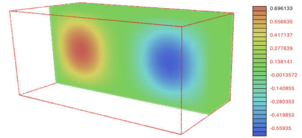
(d) final solution field
