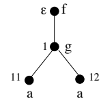
Fig. 2. f(g(a, a))
