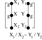
Fig. 19. Local variables?
