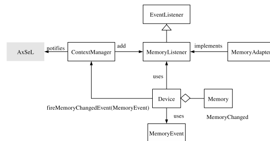
Figure 6. Écouteur abonné à la mémoire du terminal
