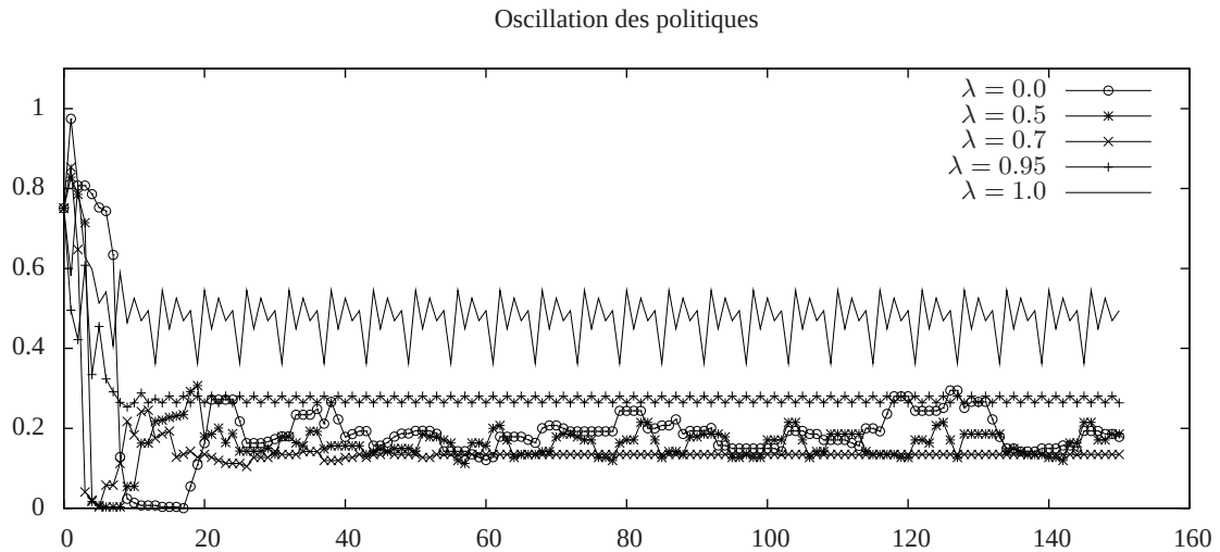
FIGURE 9 – Chaîne d'états. Évolution de \|Q^{\pi_k} - Q^*\|_{\infty} , distance entre la valeur de la politique courante et la valeur optimale, pour l'expérience de la figure 8 avec la méthode PF.
