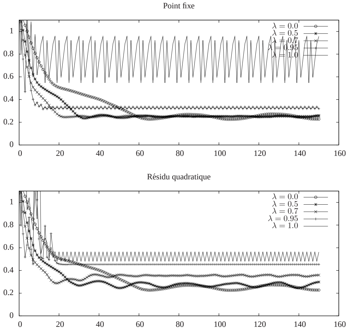
FIGURE 8 – Evolution au cours des itérations de \|\hat{Q}_k - Q^*\|_\infty , distance entre la fonction de valeur approximative courante et la fonction de valeur optimale, pour plusieurs valeurs de \lambda . Fonctions de base gaussiennes. \gamma = 0.95 . Moyenne de 10 exécutions, les exécutions utilisant des ensembles d'épisodes de 200 échantillons. Haut : méthode PF. Bas : méthode RQ.
