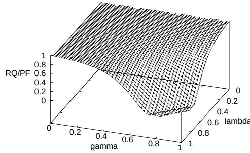
FIGURE 6 – \frac{|\alpha_{RQ}|}{|\alpha_{PF}|} en fonction de \lambda et \gamma .
