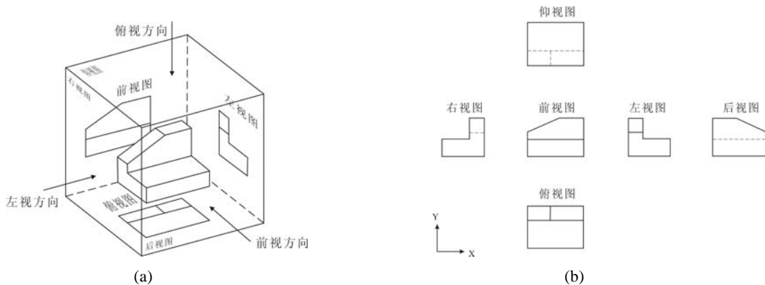
图 1 第一角投影的基本视图
