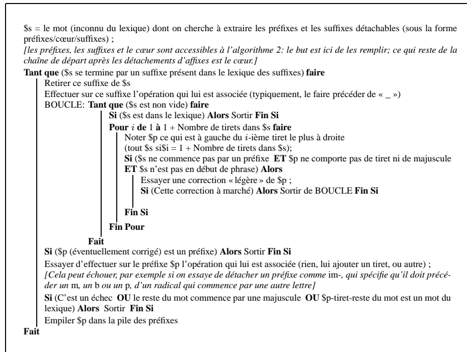
Algorithme 4: Heuristique simplifiée pour TEXT2DAG: identification des affixes.
