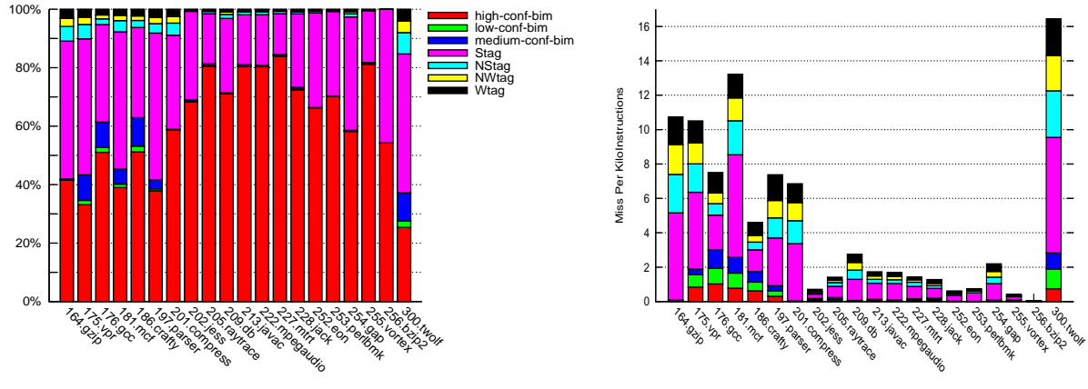
16Kbits predictor
