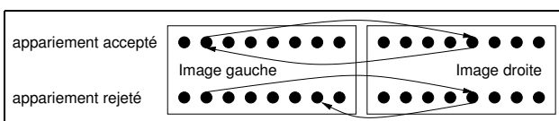
FIG. 6 – Vérification bidirectionnelle.
