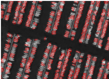
(a) Résultat de simulation d'une configuration d'objets à la dernière itération de l'algorithme SEM
