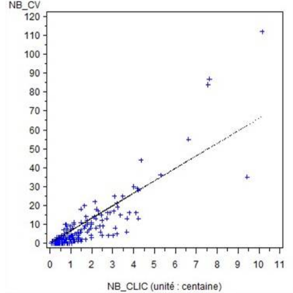
Figure 2 : NB_CV en fonction de NB_CLIC et droite de régression sans constante
