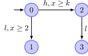
Fig. 1. Automaton A(k)
