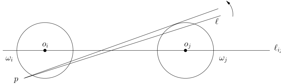
Figure 3: Lemma 3.1.
