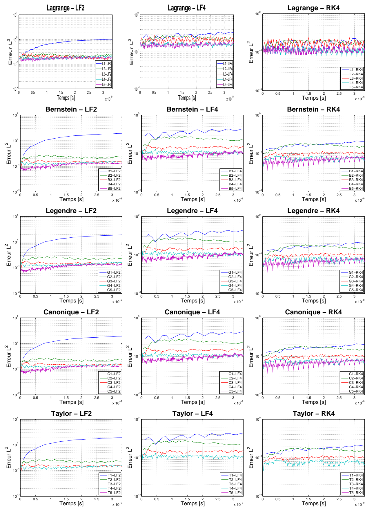
FIG. 48 – Propagation du pulse créneau Evolution temporelle de l'erreur L^2 , N=81 points
