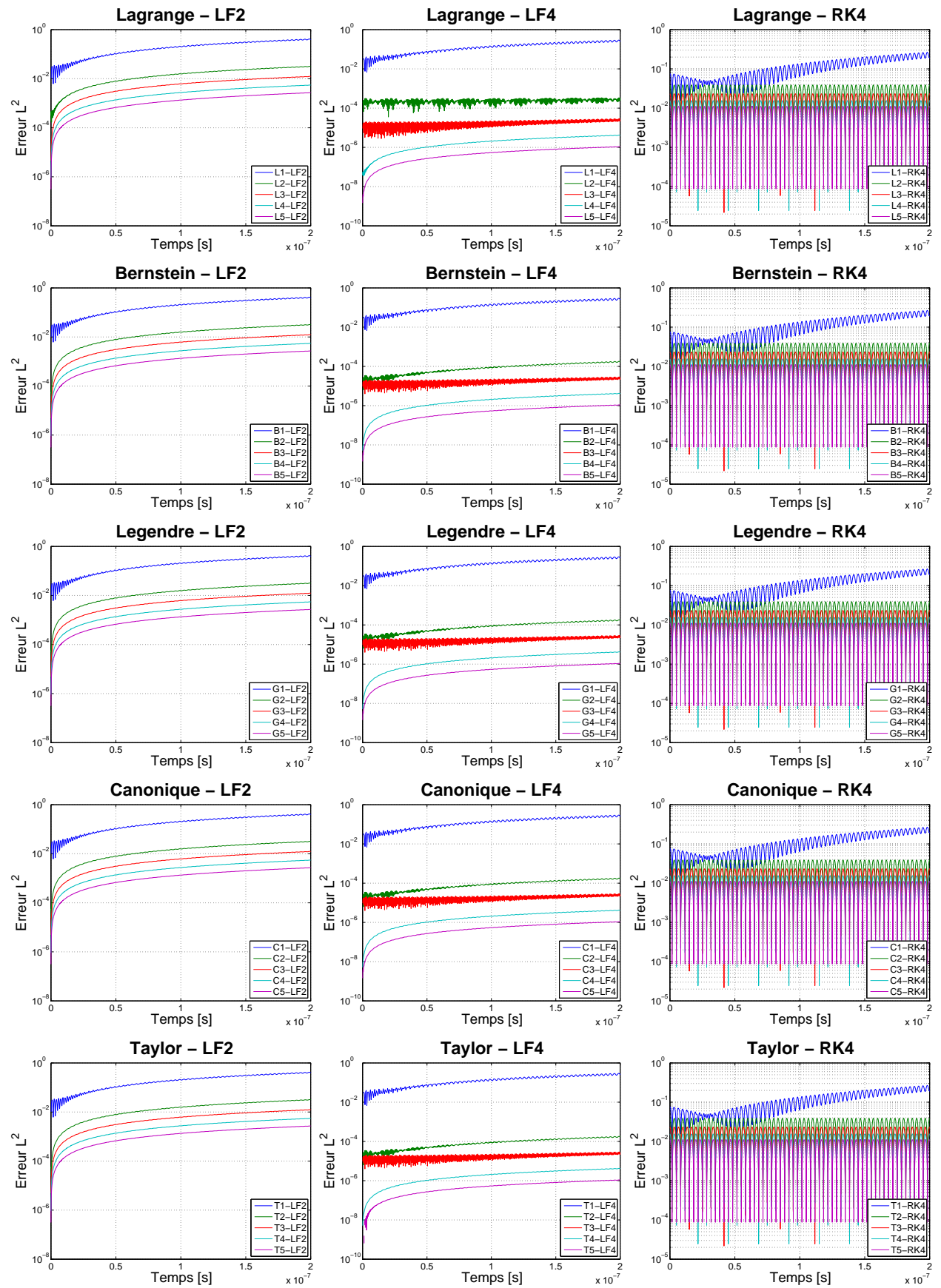
FIG. 14 – Propagation du mode fondamental Evolution temporelle de l'erreur L^2 , N=11 points
