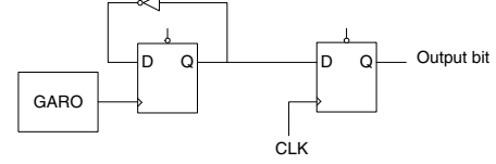
Fig. 7. GARO generator.
