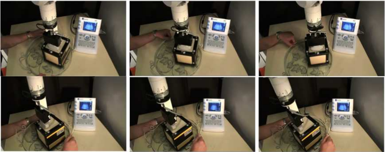
Fig. 6. Poursuite automatique d'une maquette anatomique, simulant le déplacement de tissus mous (selon 6 DDL), par une sonde échographique 2D embarquée sur un robot. L'asservissement visuel utilise uniquement le bruit de "speckle" contenu dans l'image échographique pour réaliser la tâche
