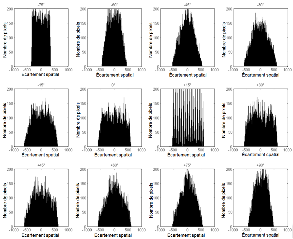
FIGURE 8. Quelques histogrammes de projection du document de la figure 6.
