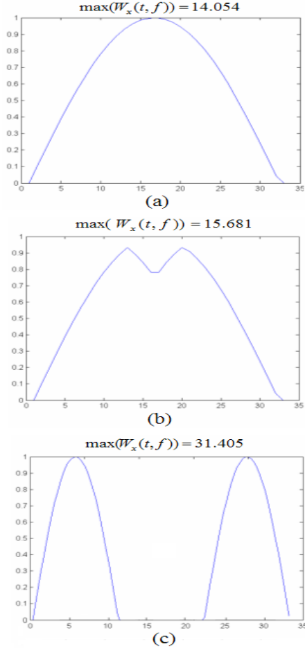
FIGURE 5. Exemples de valeurs maximales de la distribution de Wigner-Ville obtenues pour différents histogrammes de projection.
