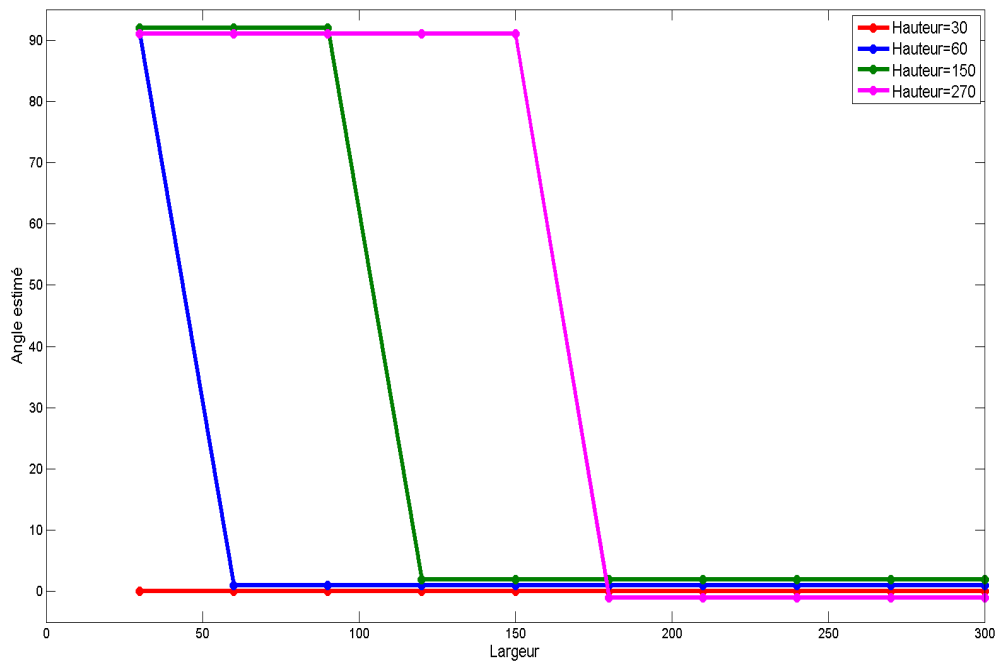
FIGURE 11. Évolution de l'estimation de l'angle d'inclinaison du document de la figure 9 en fonction de la largeur du document, pour quatre valeurs différentes de la hauteur. L'inclinaison est estimée en utilisant la distribution de Wigner-Ville.
