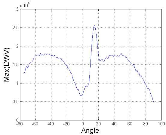
FIGURE 7. Courbe du maximum de la distribution de Wigner-Ville de la racine carrée des histogrammes de projection du document de la figure 6, en fonction de l'angle de projection.
