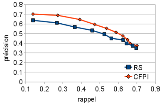
Fig. 9. Résultats obtenus avec le CFPI et la \mathcal{R} -signature pour des requêtes avec des symboles incomplets.
