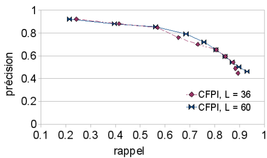
Fig. 6. Précision/rappel avec descripteurs CFPI (dimension L = 36, 60)
