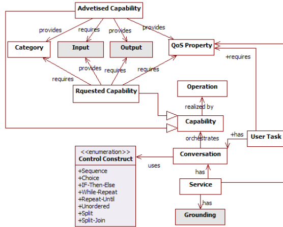
Fig. 4. COCOA-L
