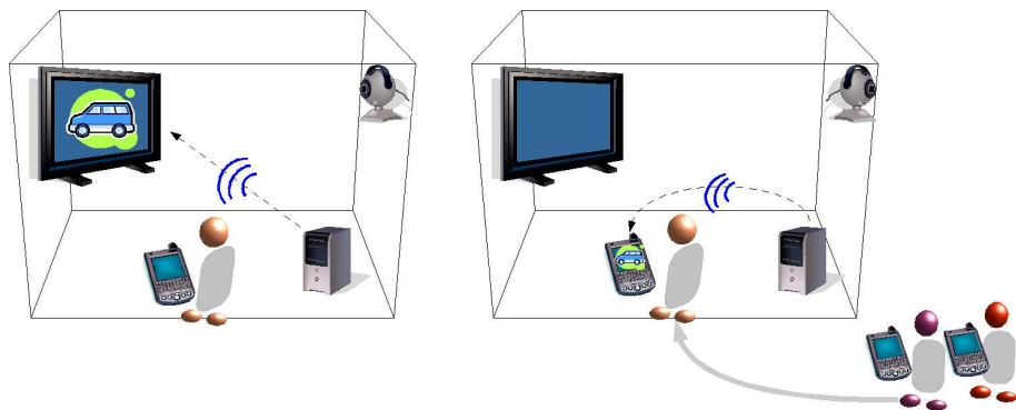
Fig. 1. Scenario
