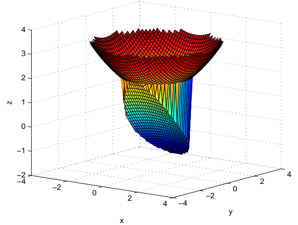
FIG. 6 – Géométrie du miroir complet combinant une surface parabolique et une surface concave pour l’observation du conducteur
