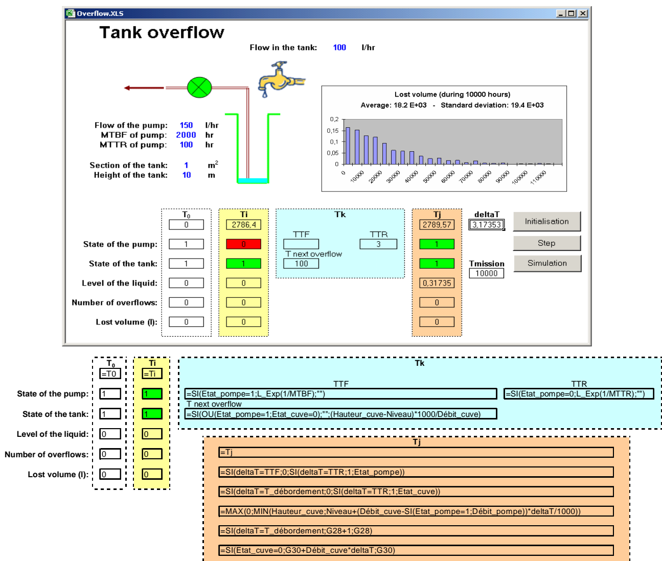
Figure 2. Débordement d'une cuve
