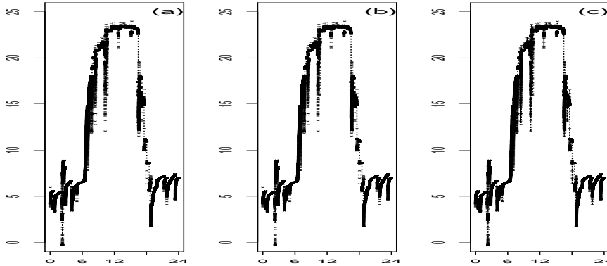
Figure 1: Représentation des estimateurs (traits en pointillés) NW (a), NWR (b) et R (c) sur les données brutes du bénitier 7 avec en abscisse le temps (h) et en ordonnée l'écartement valvaire (mm).
