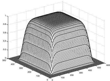
Fig. 15. Function f(u)f(v) .
