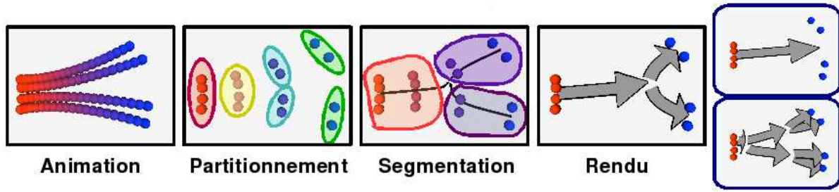
Figure 3: Aperçu de notre algorithme : nous prenons en entrée un ensemble de particules animées. Les trajectoires sont découpées par l'algorithme de Mean Shift (section 3.2), segmentées (section 4.1), avant d'être affichées sous forme de flèches représentatives du mouvement (section 3.3). L'utilisateur peut faire varier l'échelle de la visualisation, obtenant ainsi soit une indication globale du mouvement (en haut à droite) soit un rendu plus détaillé (bas droite).
