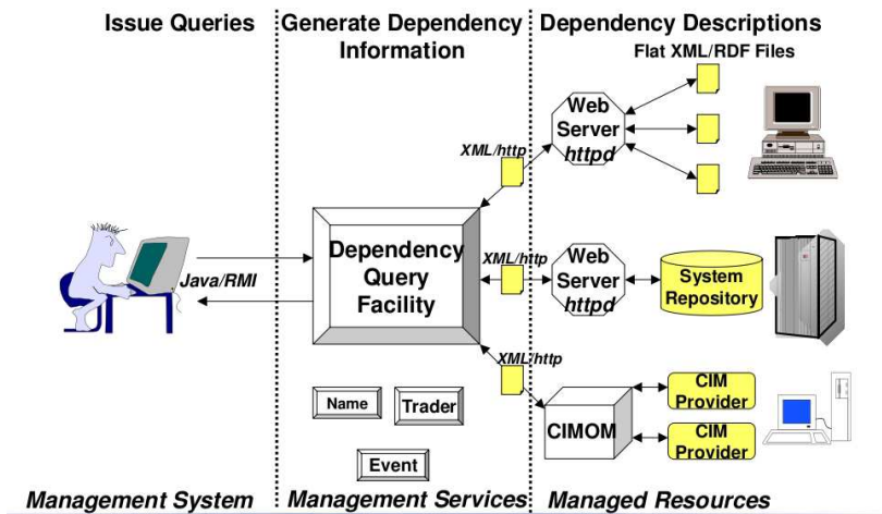
FIG. 1.12 – Architecture du système de dépendances[5]
