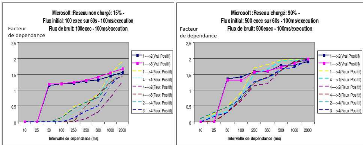
FIG. 3.2 – Effet de l'intervalle de dépendance
