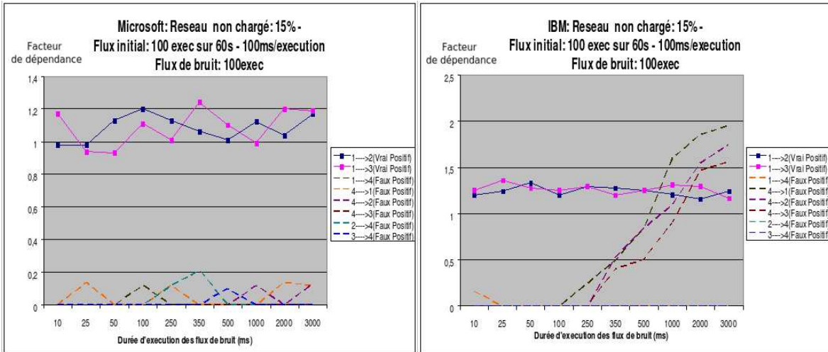
FIG. 3.3 – L’effet de la durée d’exécution des flux de bruit : sur un réseau non chargé
