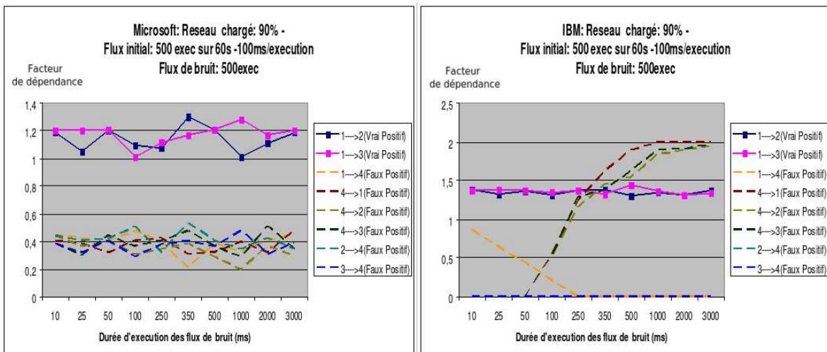
FIG. 3.4 – L’effet de la durée d’exécution des flux de bruit : sur un réseau chargé
