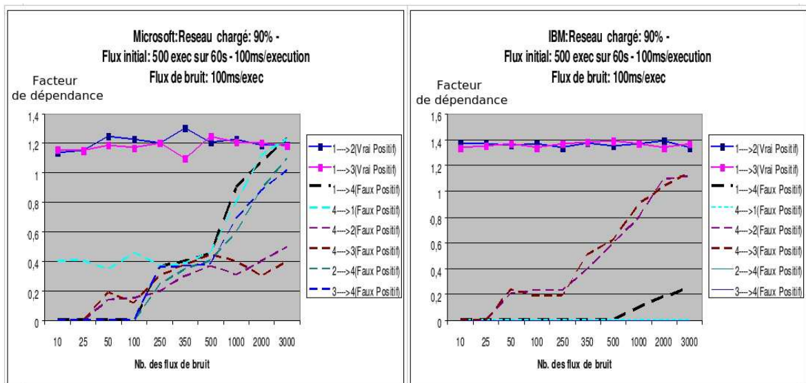
FIG. 3.6 – L'effet du nombre des flux de bruit sur un réseau chargé
