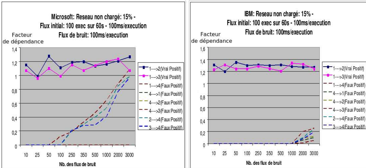
FIG. 3.5 – L'effet du nombre des flux de bruit sur un réseau non chargé
