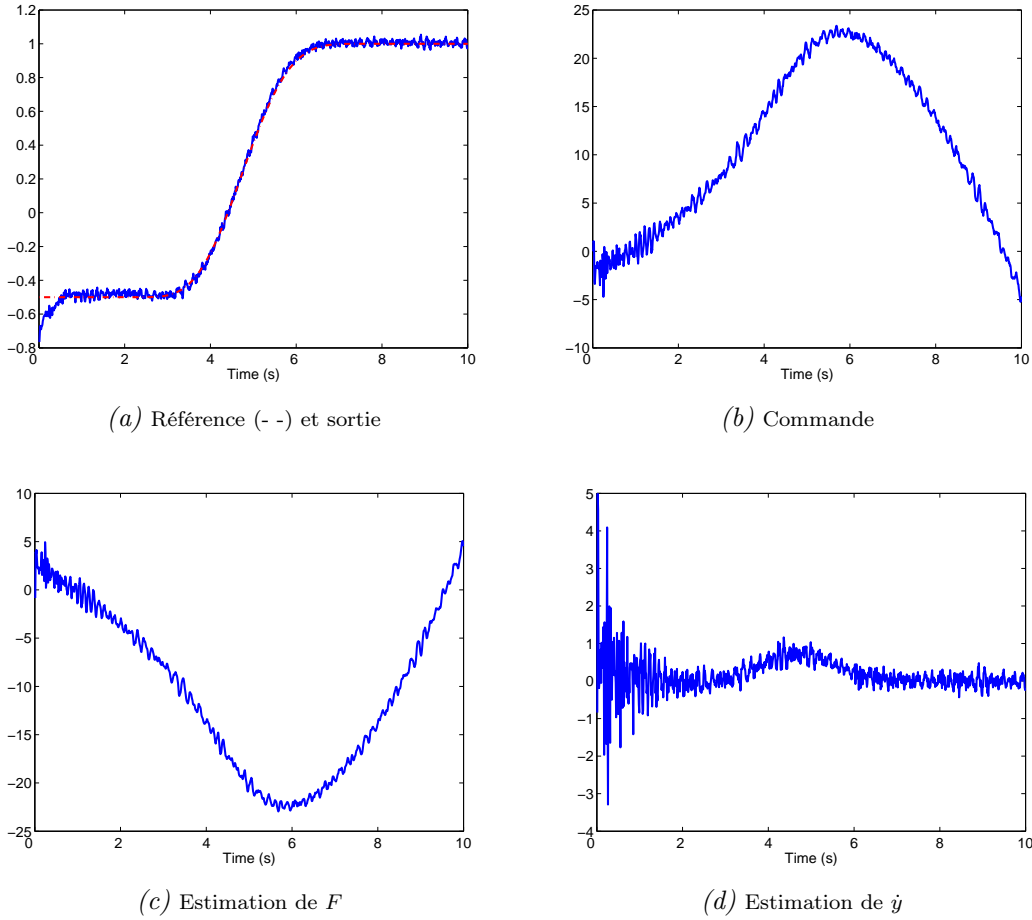
Fig. 4: Système linéaire monovariante à large spectre
