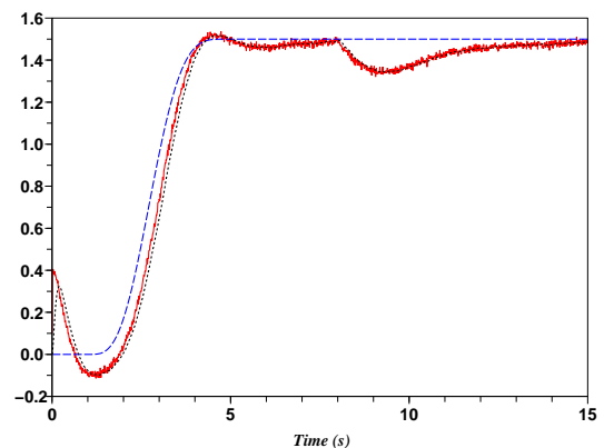
(d) Sortie (-); référence (- -); sortie débruitée (. .)
