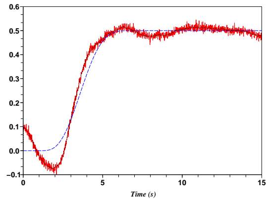
(d) i-PID : sortie (-), référence (- -); sortie débruitée (. .)
