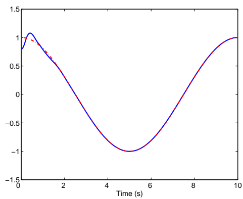
(a) Référence (- -) ; sortie
