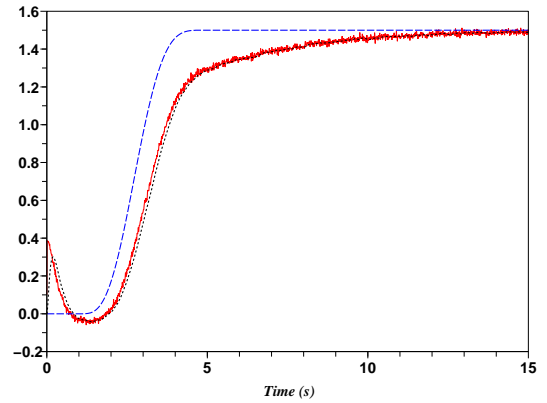
(d) Sortie (-); référence (- -); sortie débruitée (. .)
