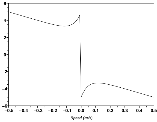
(a) Loi du frottement
