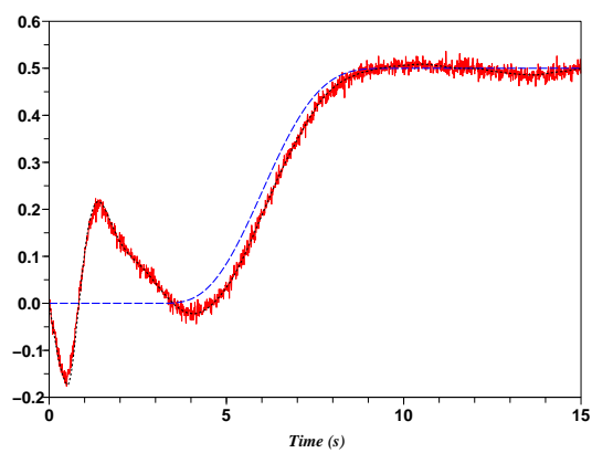
(e) Sortie (-); référence (- -); sortie débruitée (. .)
