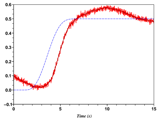
(h) PID sans platitude : sortie (-), référence (- -), sortie débruitée (. .)
