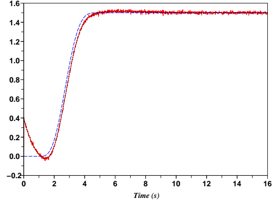
(b) Sortie (-); référence (- -); sortie débruitée (. .)
