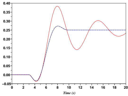
(a) u (-); u^* (- -)
