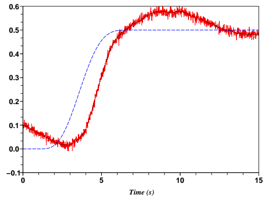
(f) Platitude + PID classique : sortie (-), référence (- -), sortie débruitée (. .)
