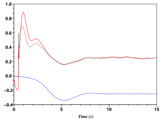
(d) u (-); u^* (- -); u_{\text{pert}}^* (. .)
