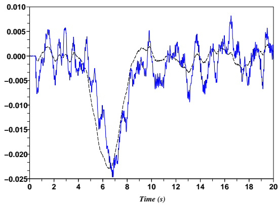
(c) Perturbation (- -); perturbation estimée (-)
