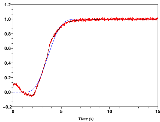
(c) Sortie (-); référence (- -); sortie débruitée (. .)
