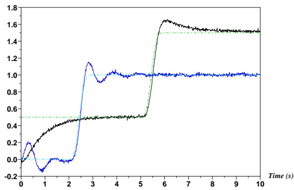
(a) i-PID : références (- -) et sorties
