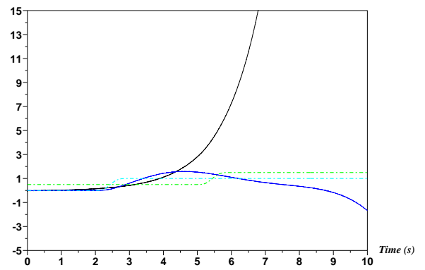
(b) PID : références (- -) et sorties
