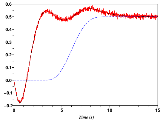
(b) Sortie (-); référence (- -); sortie débruitée (. .)
