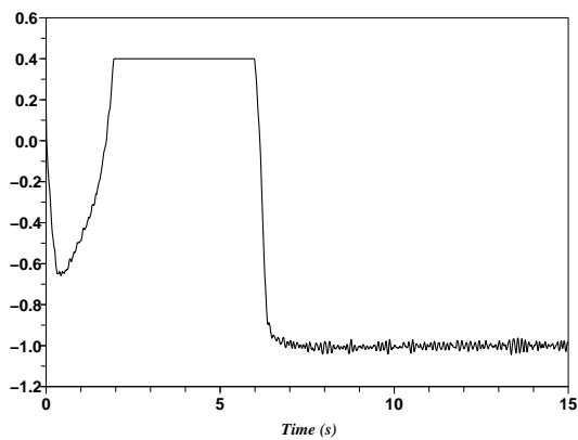
Fig. 9: Système non linéaire instable : commande saturée avec anti-emballement
