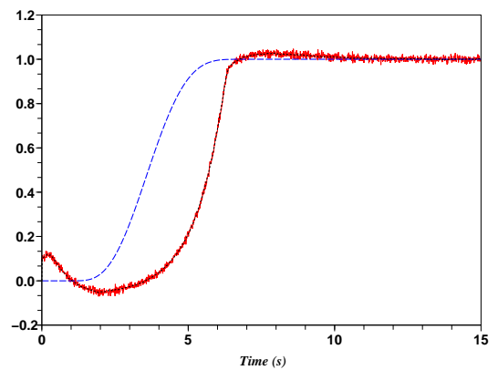
Fig. 9: Système non linéaire instable : commande saturée avec anti-emballement
