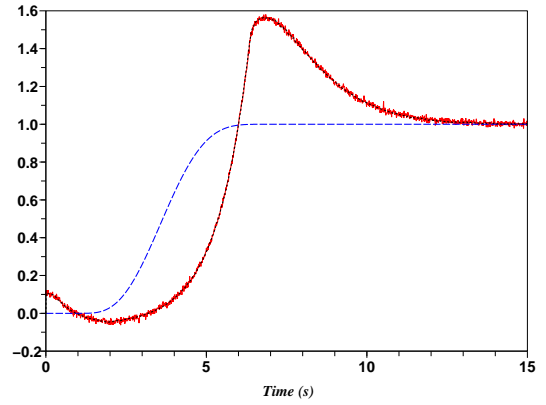
Fig. 8: Système non linéaire instable : commande saturée sans anti-emballement
