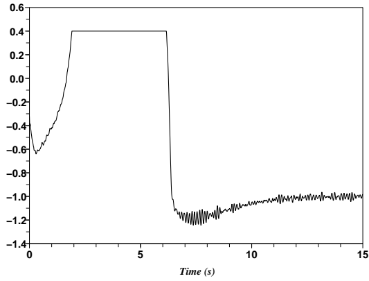
Fig. 8: Système non linéaire instable : commande saturée sans anti-emballement
