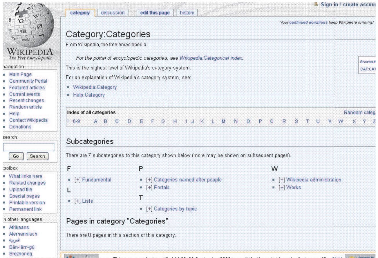
FIG. 3 – la catégorie des catégories.
