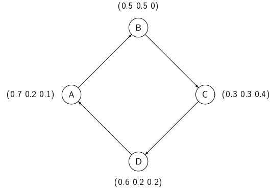
FIG. 5. Un cas de coupes de cycles pour les sommets A et C (première couleur) et les sommets B et D (troisième couleur).
