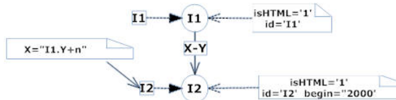
Figure 16: La représentation de l'ordonnement de synchrobase
