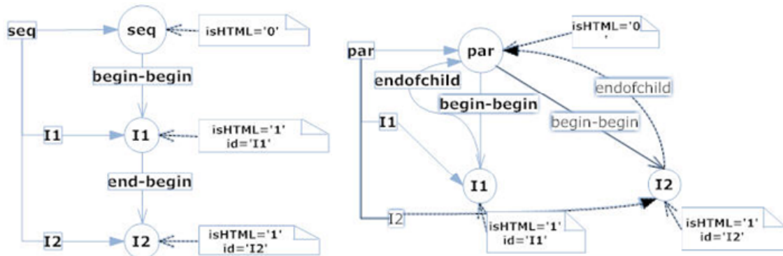
Figure 17: La représentation d'ordonnement de (a) conteneur "seq" et (b) conteneur "par"
