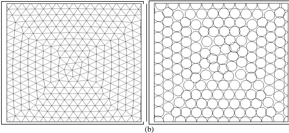
Figure 27. La structure granulaire à droite et la triangulation à gauche, a) avant, (b) après l'application de l'algorithme du lissage.
