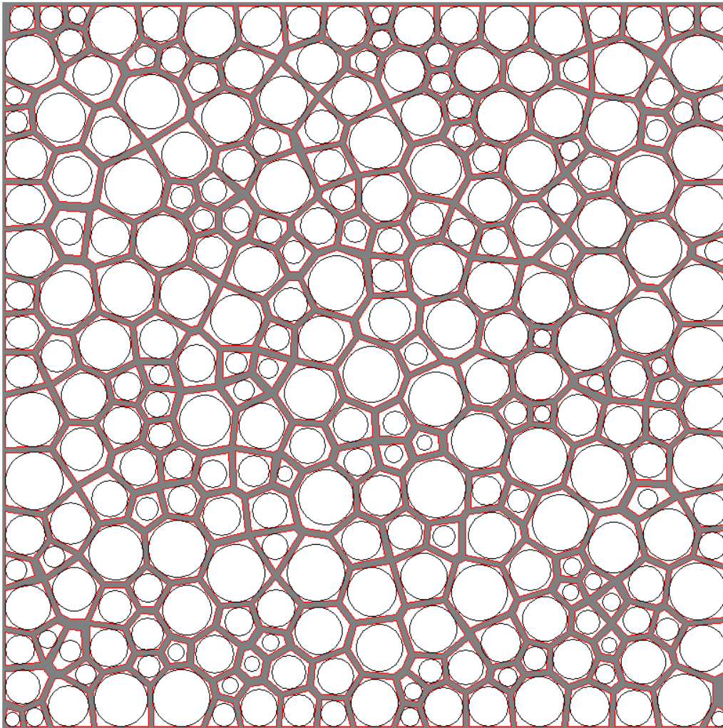
Figure 41. Rétrécissement des cellules (en rouge) et dissociation des joints de grains (bandes en gris).
