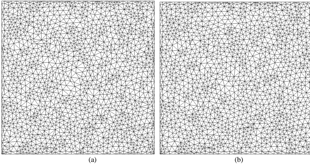
Figure 37. Structure granulaire et triangulation correspondante, a) avant, b) après l'application de notre algorithme d'optimisation dans le cas de rayons variables.
