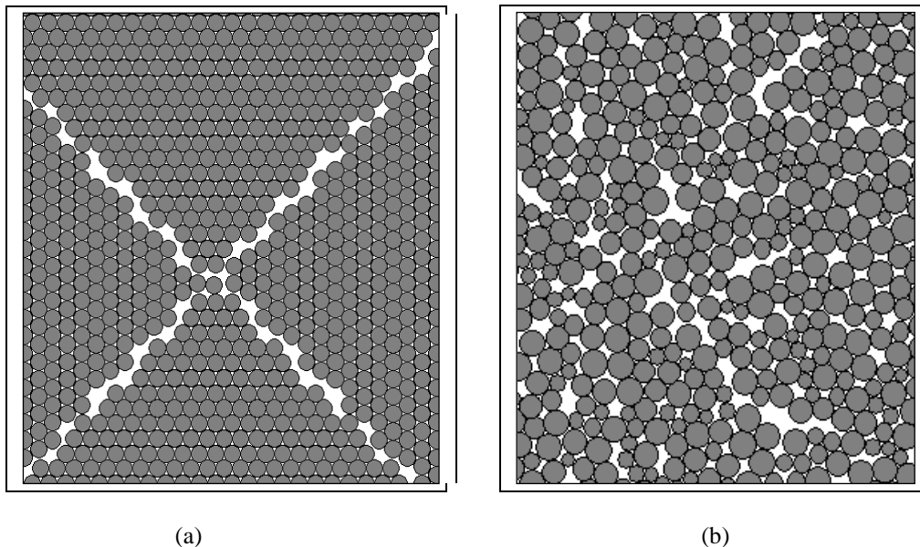
Figure 24. Extraits de structures générées par notre algorithme de remplissage, (a) cas d'un rayon fixe, (b) cas de rayons variables.
