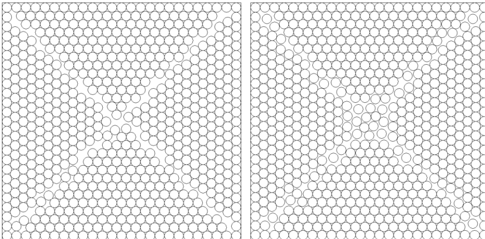
Figure 28. La structure granulaire : à gauche avant optimisation et à droite après l'application de l'algorithme du lissage sous contrainte.
