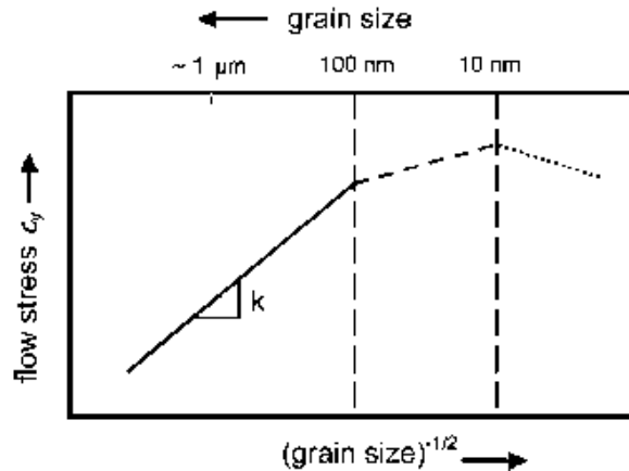
Figure 1. Variation d'une propriété physique (ici la limite élastique) en fonction de la taille moyenne des grains.
