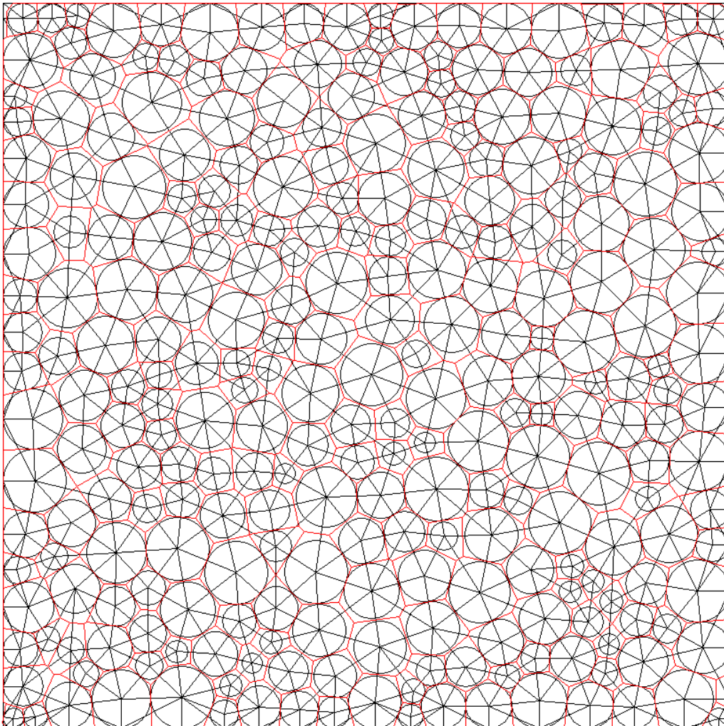
Figure 39. Triangulation Delaunay pondérée (triangles en noir) et son dual le diagramme de Laguerre (en rouge).
