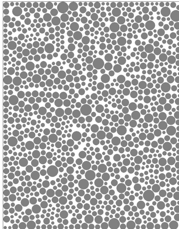
Figure 23. La structure générée du fer pur nanostructuré : les disques représentent les grains et les espaces entre ceux-ci les joints de grains.
