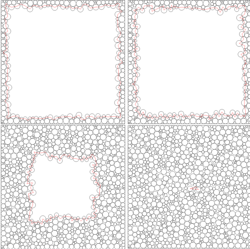
Figure 14. Illustration de quelques étapes de remplissage réalisé par notre algorithme.
