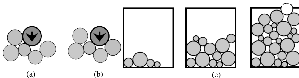
Figure 10. (a) Position instable. (b) Position stable. (c) Exemple d'un remplissage par la méthode de droppage.
