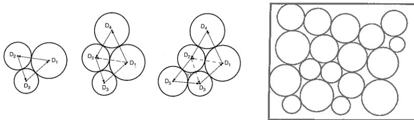
Figure 12. À gauche : illustration de la méthode du front fermé. À droite : un exemple de remplissage avec cette méthode.
