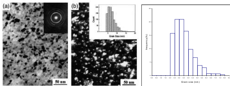
Figure 3. La structure observée par microscopie d'un échantillon de fer pur nanostructuré. Les histogrammes représentent la distribution (fréquences en fonction des rayons) pour cet exemple.
