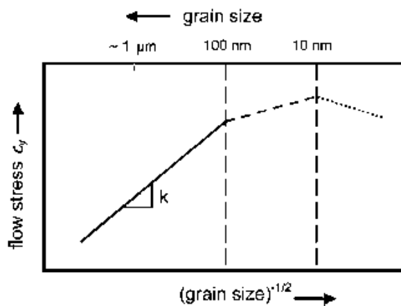
Figure 2. Variation d'une propriété physique (ici la limite élastique) en fonction de la taille moyenne des grains.
