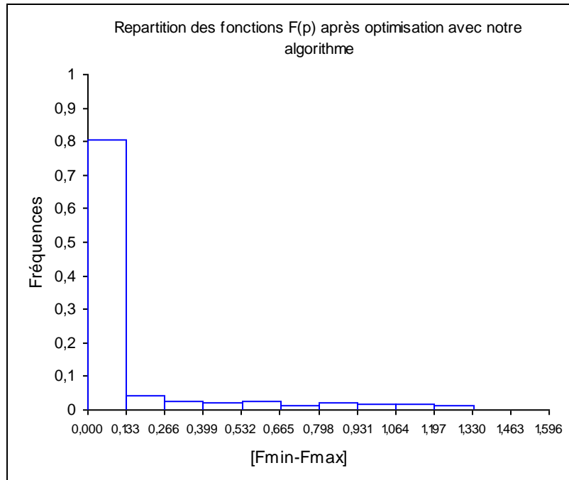
Figure 37. Histogrammes après optimisation avec notre algorithme.
