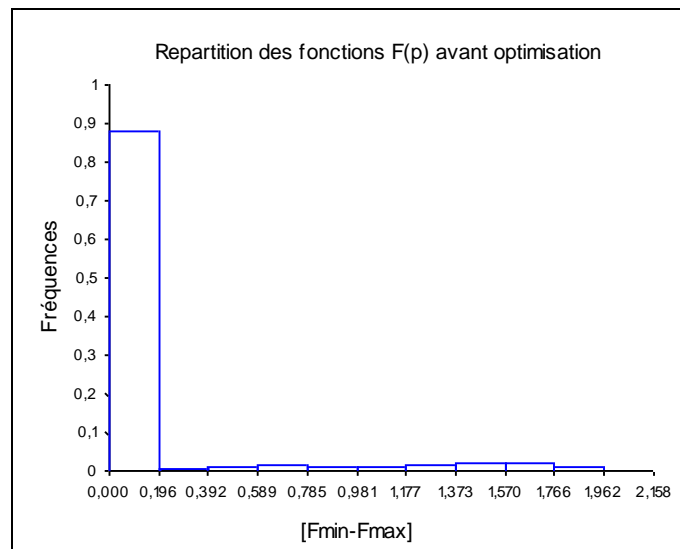
Figure 30. Histogrammes avant optimisation.
