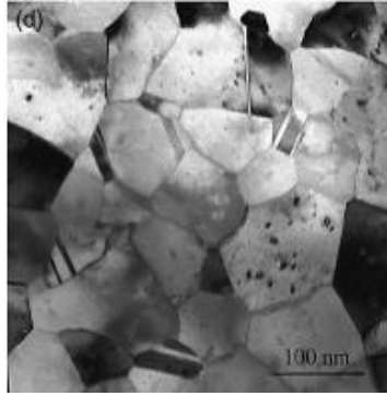
Figure 3. Grains en forme de cellules de Laguerre observées par microscopie.
