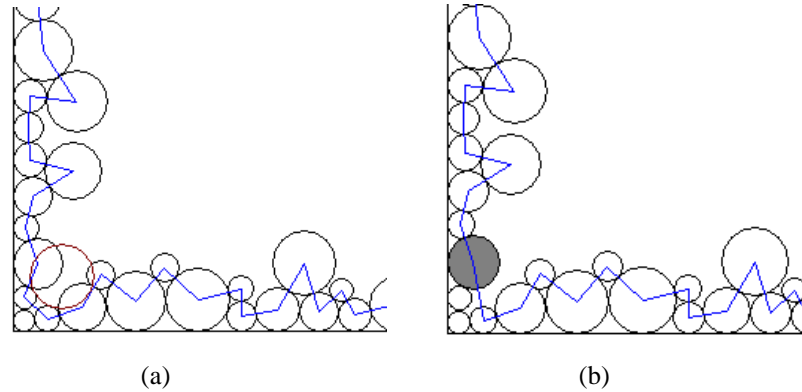
Figure 22. (a) Détection des conflits entre le nouveau disque (en rouge) et des disques existants lorsque le premier segment actif du front est sélectionné (cas défavorable de l'algorithme 1). (b) Le disque plein (en gris) est le disque p_k du critère de distance de l'équation 5, et le front est actualisé en désactivant deux segments existants et en ajoutant un nouveau.
