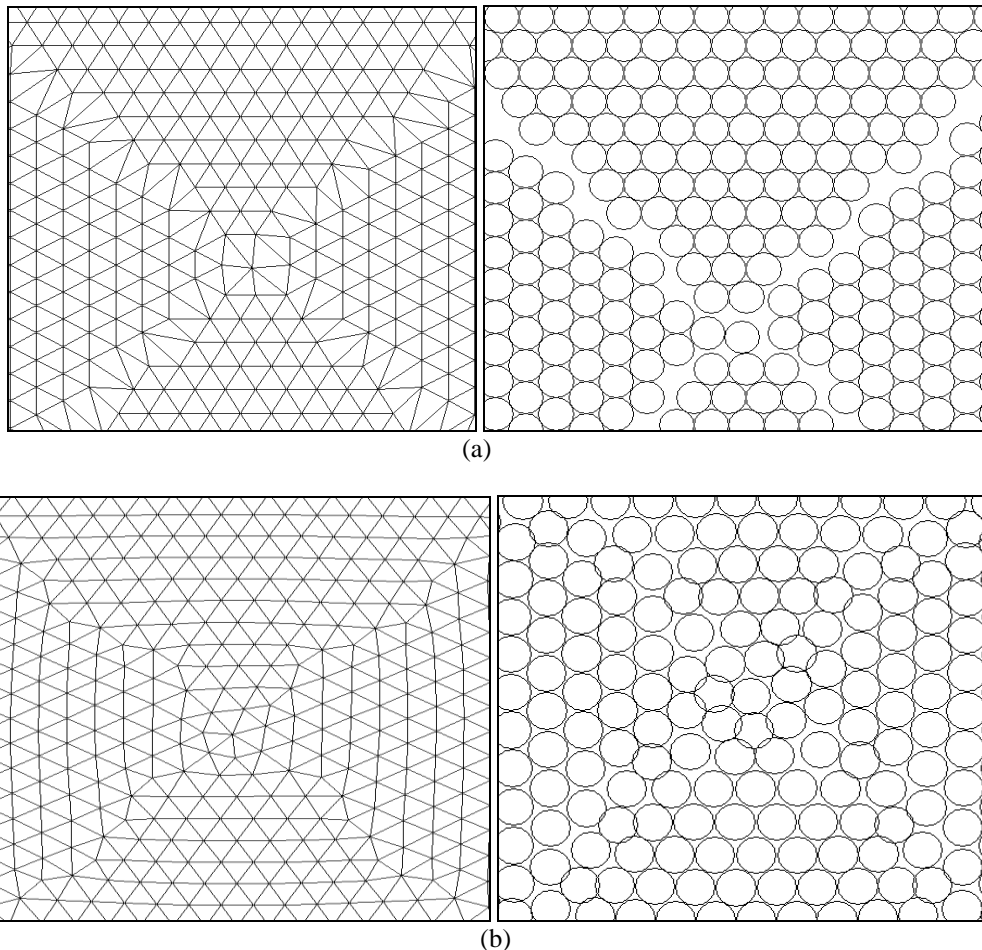
Figure 28. La structure granulaire à droite et la triangulation à gauche, a) avant, (b) après l'application de l'algorithme du lissage.
