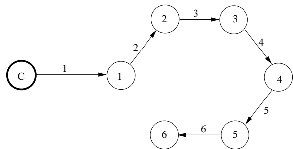
Fig. 2. L'approche adaptative : le client C accède à un quorum en contactant chaque serveur du quorum tour-à-tour. Les opérations sont exécutées en temps O(q) .
