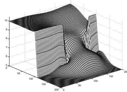
(e) à t = 7.4s FIG. 6 – Rupture partielle de barrage
