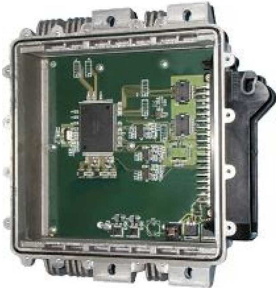
Figure 2. Calculateur E 35.
