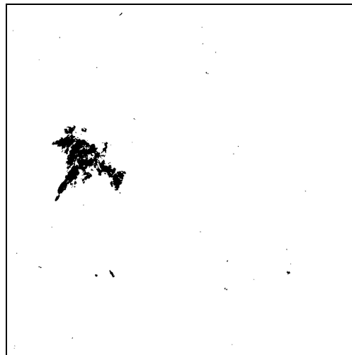
(d) SVM
