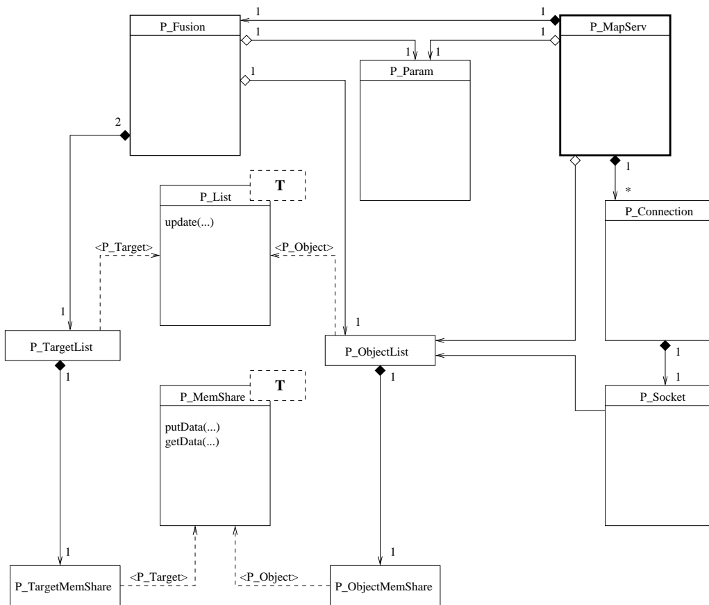
FIG. 5.20 – Graphe de classes UML du serveur de cartes
