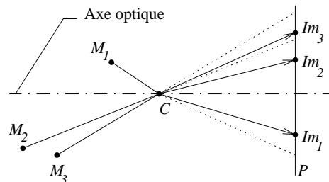
FIG. 3.6 – Incidence des rayons passant par le centre optique
