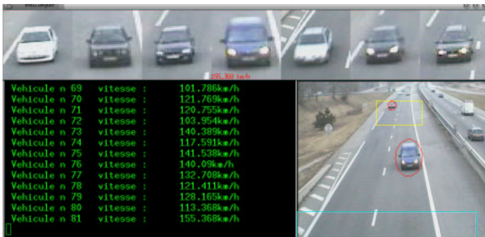
FIG. 6.9 – Ecran de visualisation d'une session de mesures de vitesse
