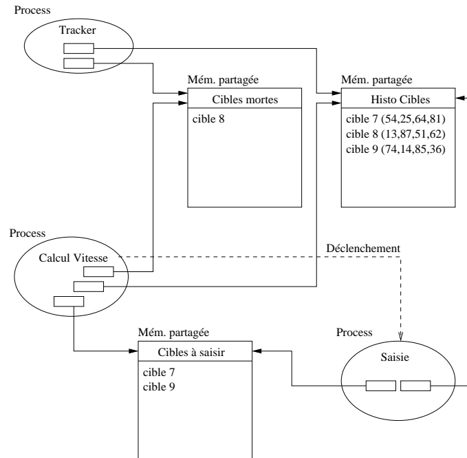
FIG. 6.3 – Architecture de l'application de mesure de vitesse
