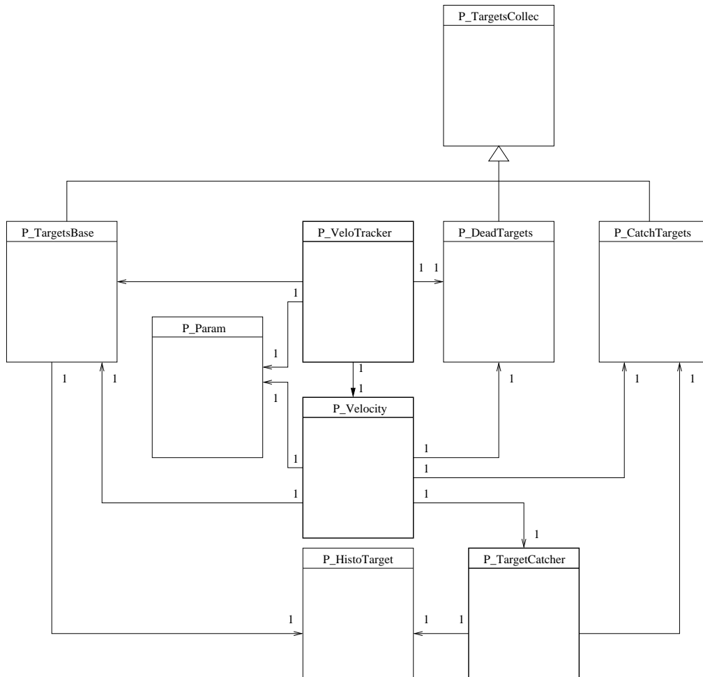
FIG. 6.4 – Diagramme UML de l'application de mesure de vitesse
