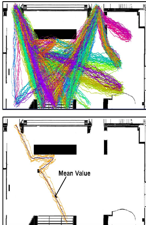
Fig. 2. Raw trajectories and a cluster obtained using DA.
