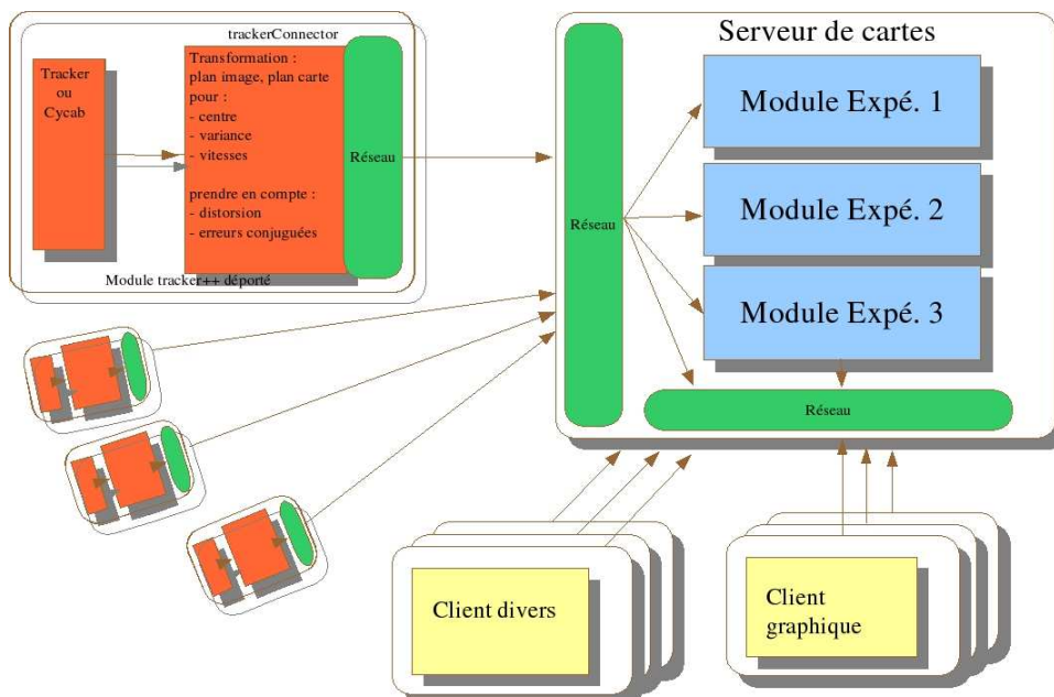
FIG. 6.2 – Nouvelle architecture
