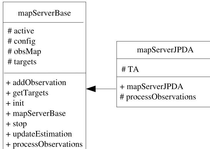
FIG. 8.37 – Classe MapServer
