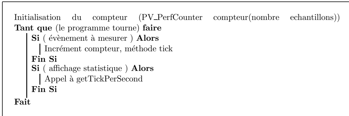
FIG. 8.21 – Algorithme du compteur de performance
