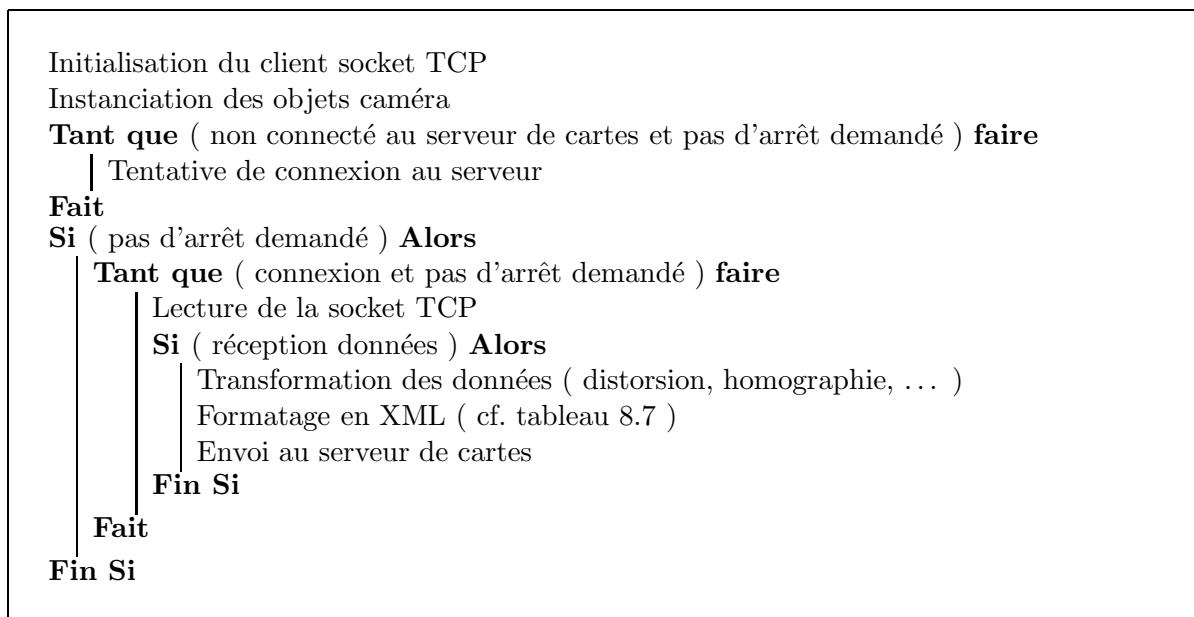
FIG. 8.28 – Algorithme du mode Primablue du trackerConnector
