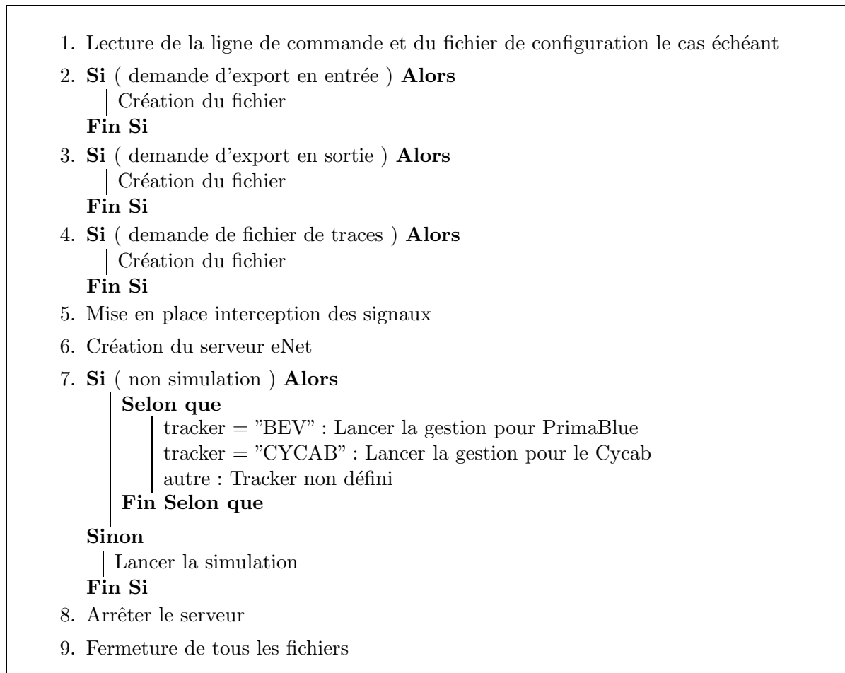
FIG. 8.23 – Algorithme global du trackerConnector
