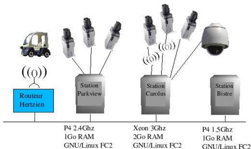
FIG. 7.1 – Infrastructure finale
