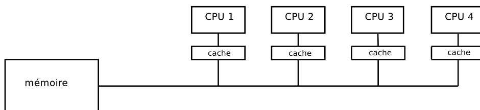
FIG. 1.1 – Machine SMP à quatre processeurs.
