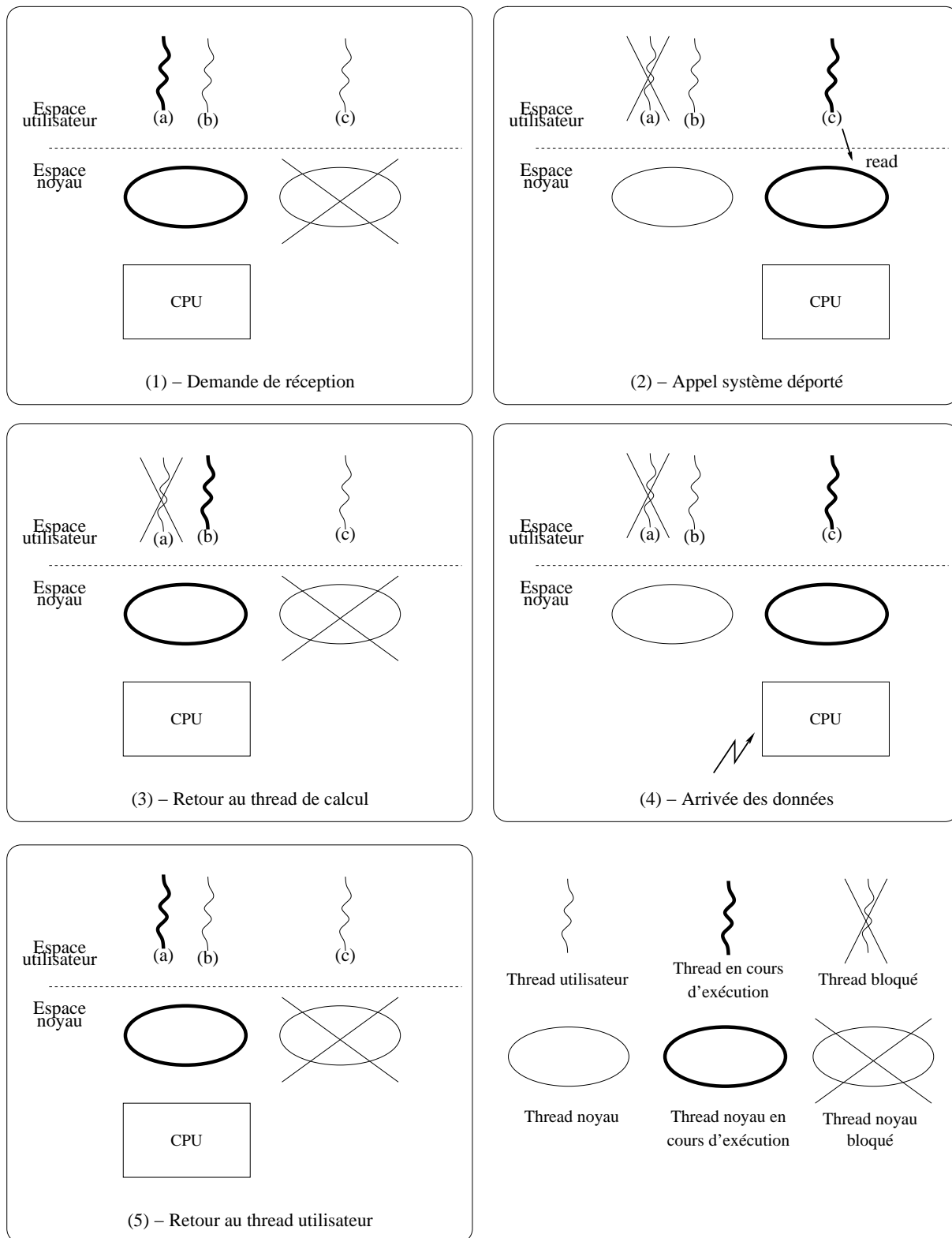
FIG. 3.2 – Déroulement d'un appel bloquant déporté
